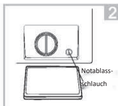
Drehen Sie den Verschluss um 90°C und ziehen Sie den Notablassschlauch heraus
