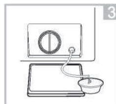
Stellen Sie eine Wanne unter und entfernen Sie die Schlauchkappe, um das Restwasser abzulassen.
